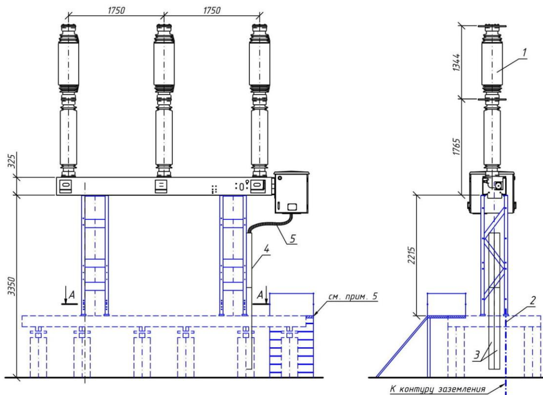
Figura 1. Amplasarea întreprupătorului pe suport mecanic zincat, prefabricat de uzina producătoare a întreprupătoarelor, conform proiectului.
